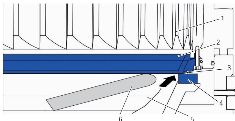
Рис. 12 Установка размера зазора с помощью измерительного щупа
