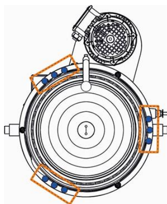
Рис. 8. Комплекты регулировочных винтов
